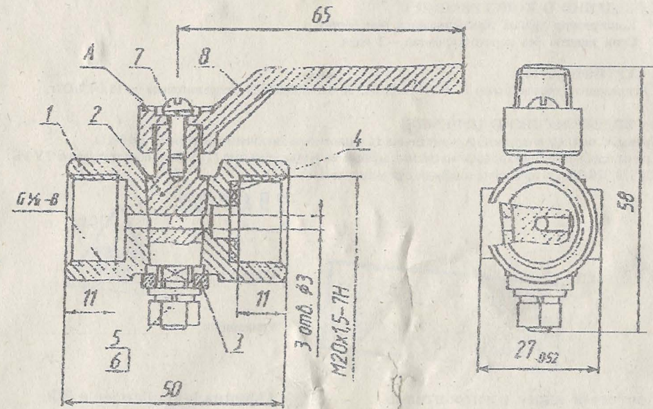
Рис. 3 – Кран КИТ 3.04.00
