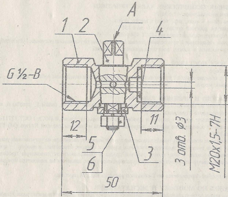
Рис. 1 – Кран КИТ 3.00.00
