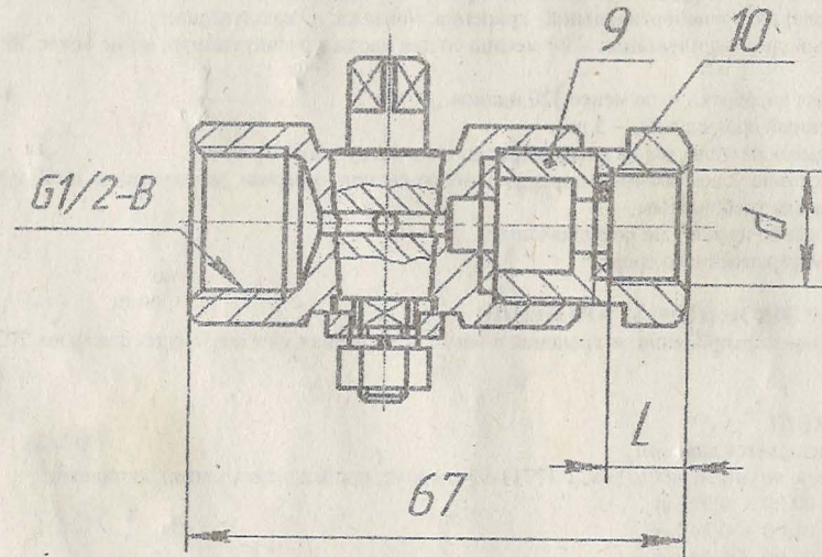
Рис. 2 – Краны КИТ 3.01.00, КИТ 3.02.00, КИТ 3.03.00
